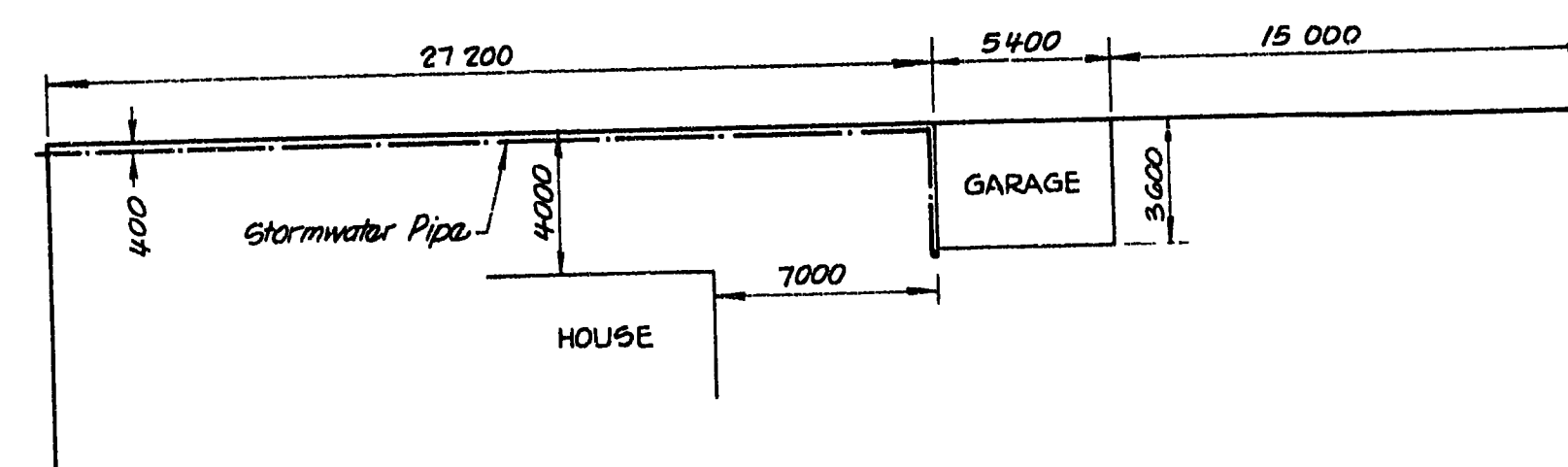
PART SITE PLAN Scale: 1:200
