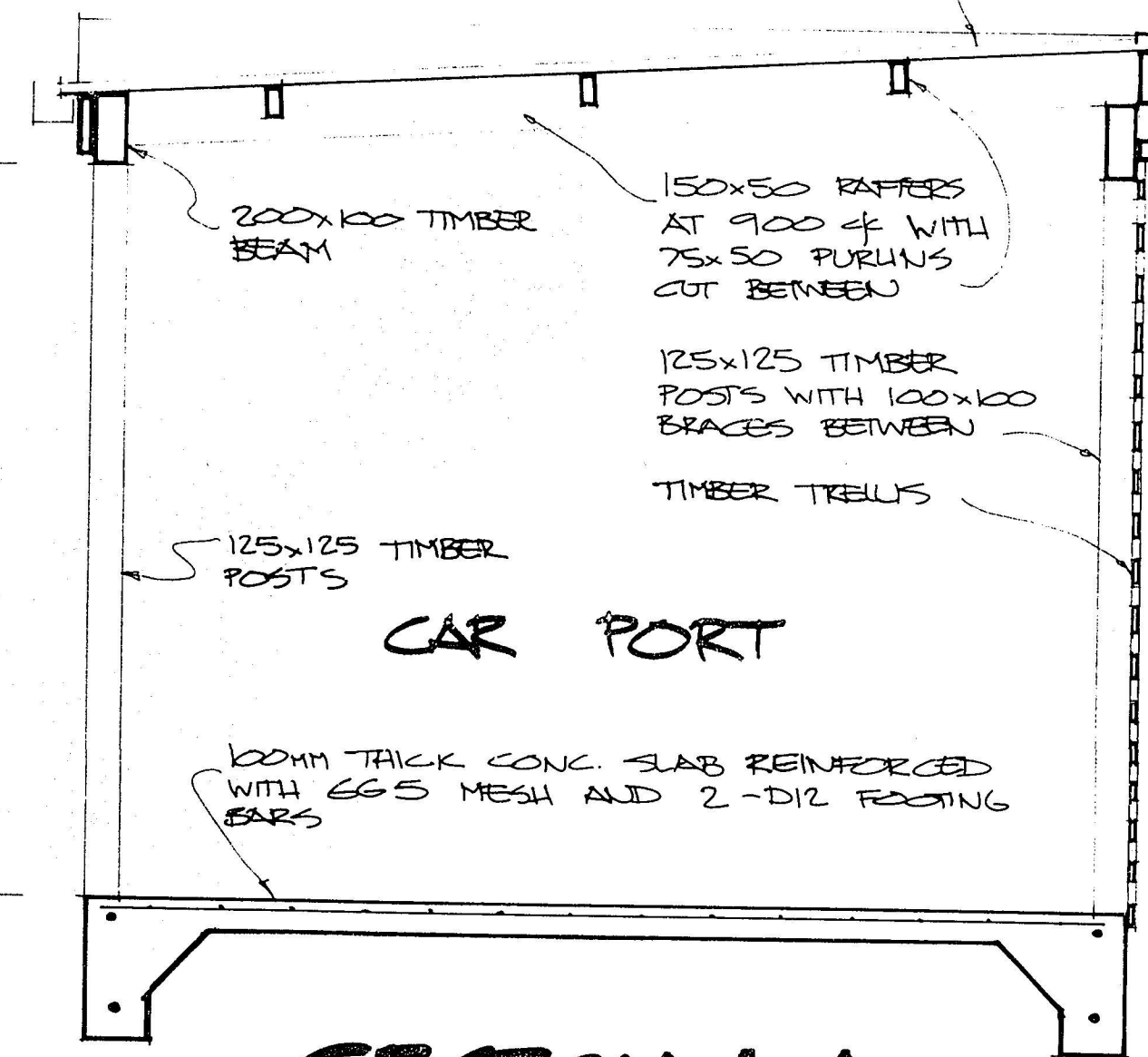
SECTION A-A 1:20
